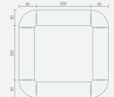
MX1646 L460 P460 H75
