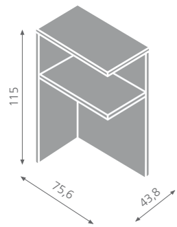
Contentitore terminale / end cabinet / armoire final / abschluss schrank / armario terminal / терминальный модуль
