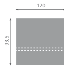
Modulo colloquio L 120 / conversation unit L 120 / réception module L 120 / besprechungsmodul B 120 / módulo conversación L 120 / прямоугольный модуль (низкий) ш.120см
