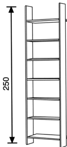
T6386 ELEMENTO DA 80 OPTIONAL UNIT, SIZE 80 L. 80 P. 25 H. 250
