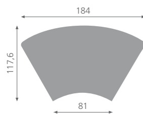
Modulo colloquio da 60° / 60° conversation unit / réception module 60° courbe / 60° besprechungsmodul / módulo conversación 60° / внутренний модуль (низкий) 60°
