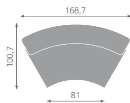
Modulo curvo da 60° interno / 60° internally curved unit / module arrondi de 60° intérieur / inneugendes modul mit 60° rundung / módulo 60° interiormente curbado / внутренний модуль 60°
