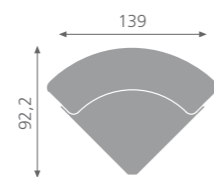
Modulo curvo da 90° interno / 90° internally curved unit / module arrondi de 90° intérieur / inneugendes modul mit 90° rundung / módulo 90° interiormente curbado / внутренний модуль 90°
