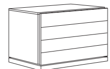
comò chest of drawers cm. L. 115 x P. 54,2 x H. 72,3
